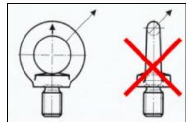
Abb. 13: Seitenzug Ringschrauben
