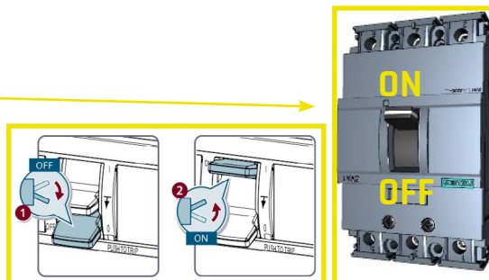
Abb. 25: Lasttrennschalter
