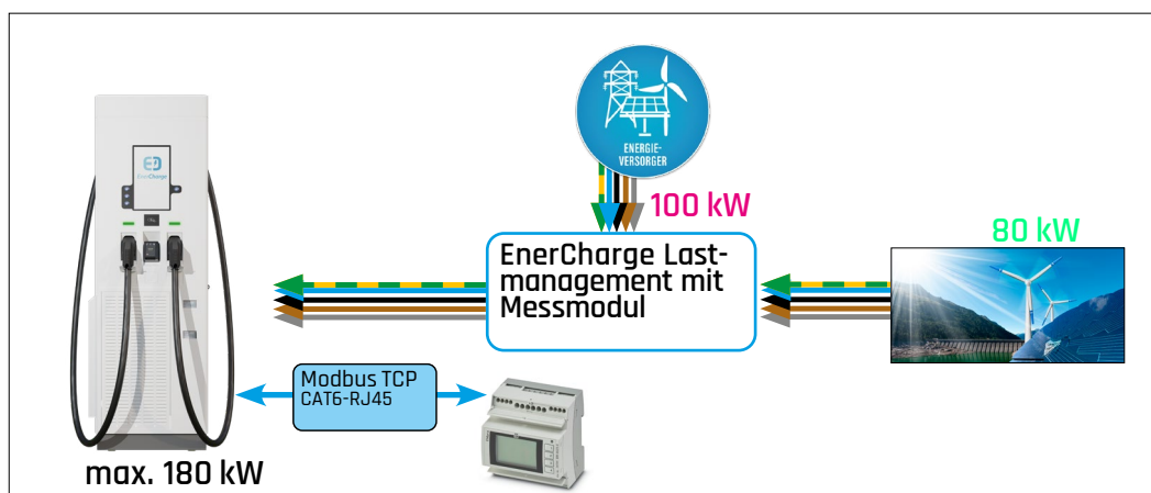
Abb. 50: Übersicht Lastmanagement Aufbau
