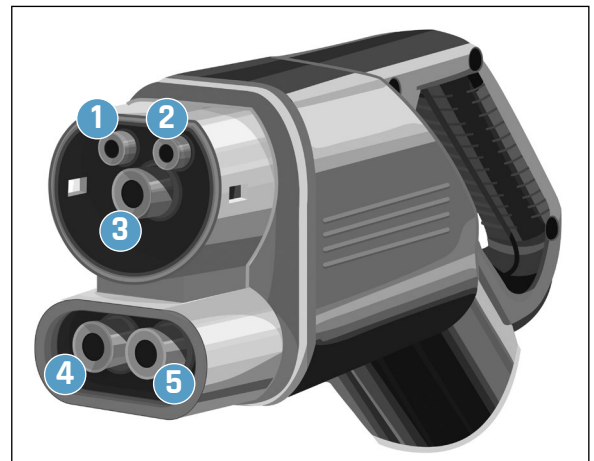
Abb. 47: CCS Ladestecker
