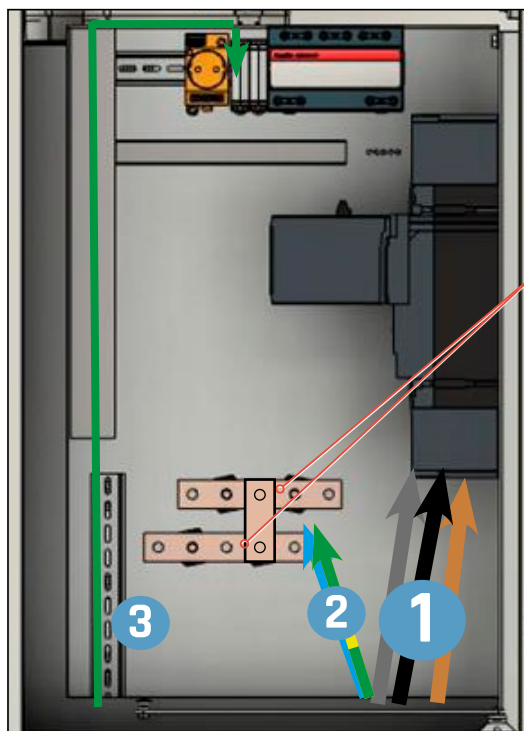
Abb. 29: Übersicht elektrische Installation ECC 320 - TN-C (4-polig)
