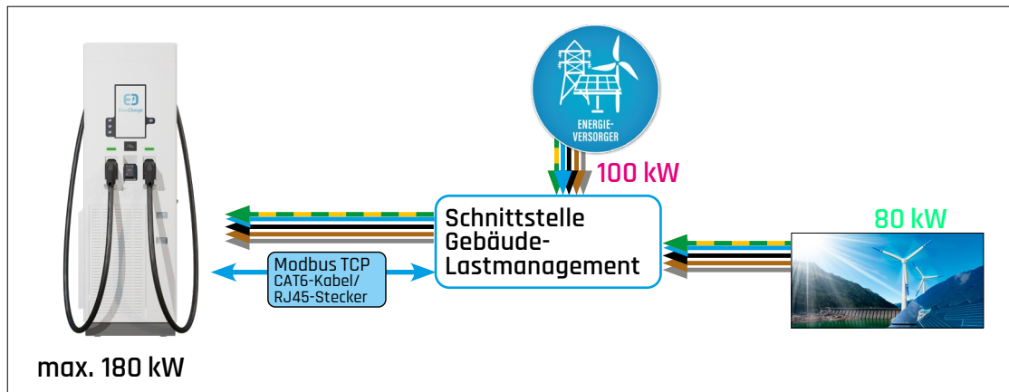
Abb. 51: Übersicht Lastmanagement Modbus Schnittstelle
