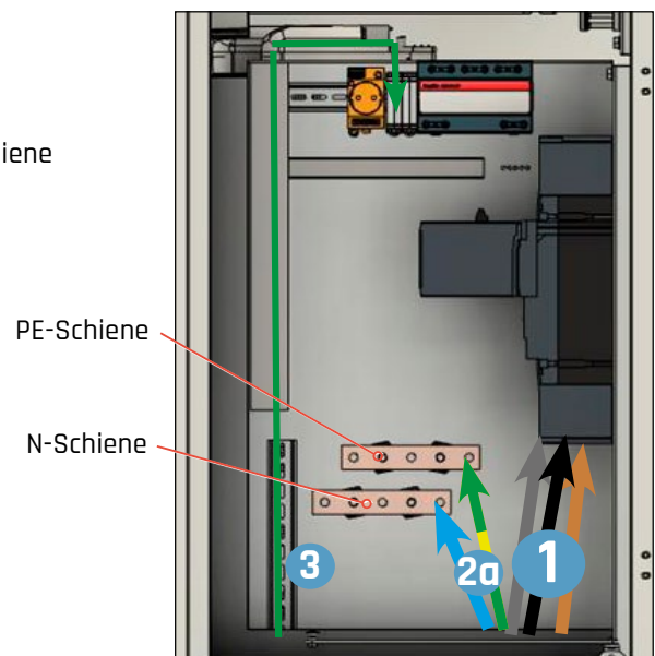
Abb. 30: Übersicht elektrische Installation ECC 320 - TN-S (5-polig)
