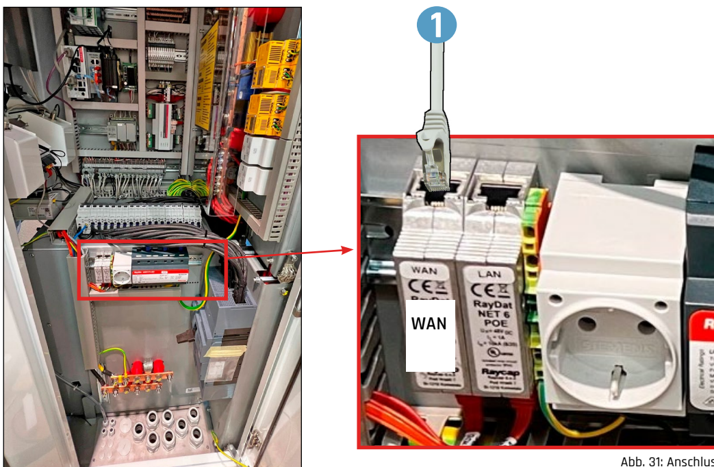
Abb. 31: Anschluss Kommunikation ECC 320
