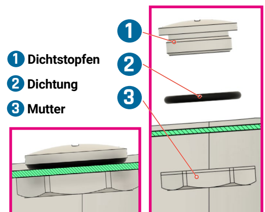
Abb. 15: Aufbau Verschraubung
