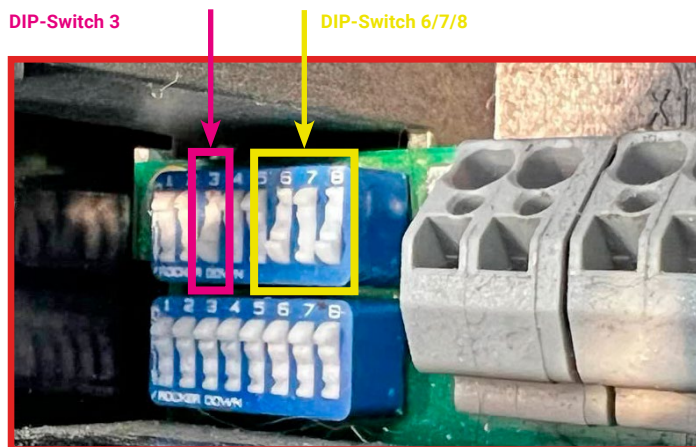
Abb. 34: Beispiel einer DIP-Switch Einstellung für 32 Ampere (22 kW)
