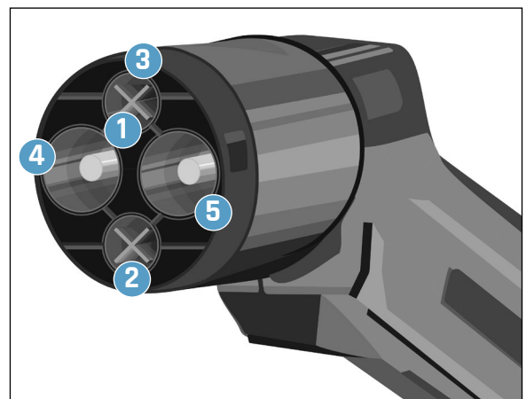
Abb. 48: CHAdeMO Ladestecker
