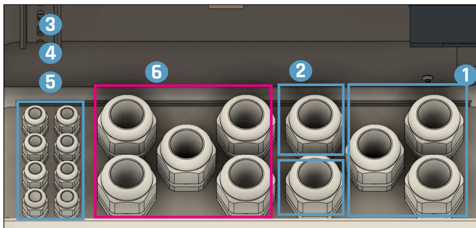
Abb. 28: Kabelbelegung Kabeldurchführungsplatte
