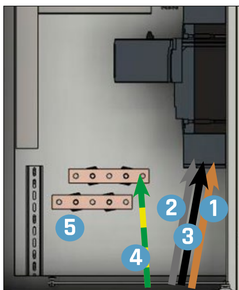
Abb. 32: Anschluss AC-Hauptzuleitung (400 V)
