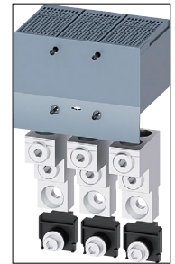
Abb. 20: Rundleiteranschlussklemme Siemens 3VA9403-0JJ23
