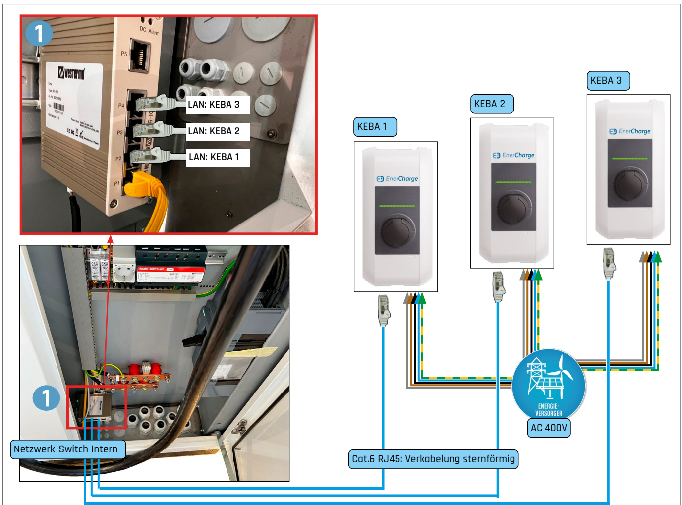
Abb. 33: Ethernet-Anschluss-Schema KEBA
