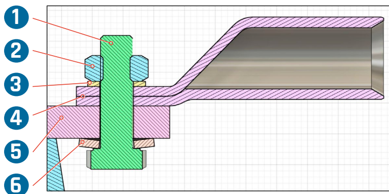
Abb. 21: Verschraubung AC-PE-N-Anschlussklemme
