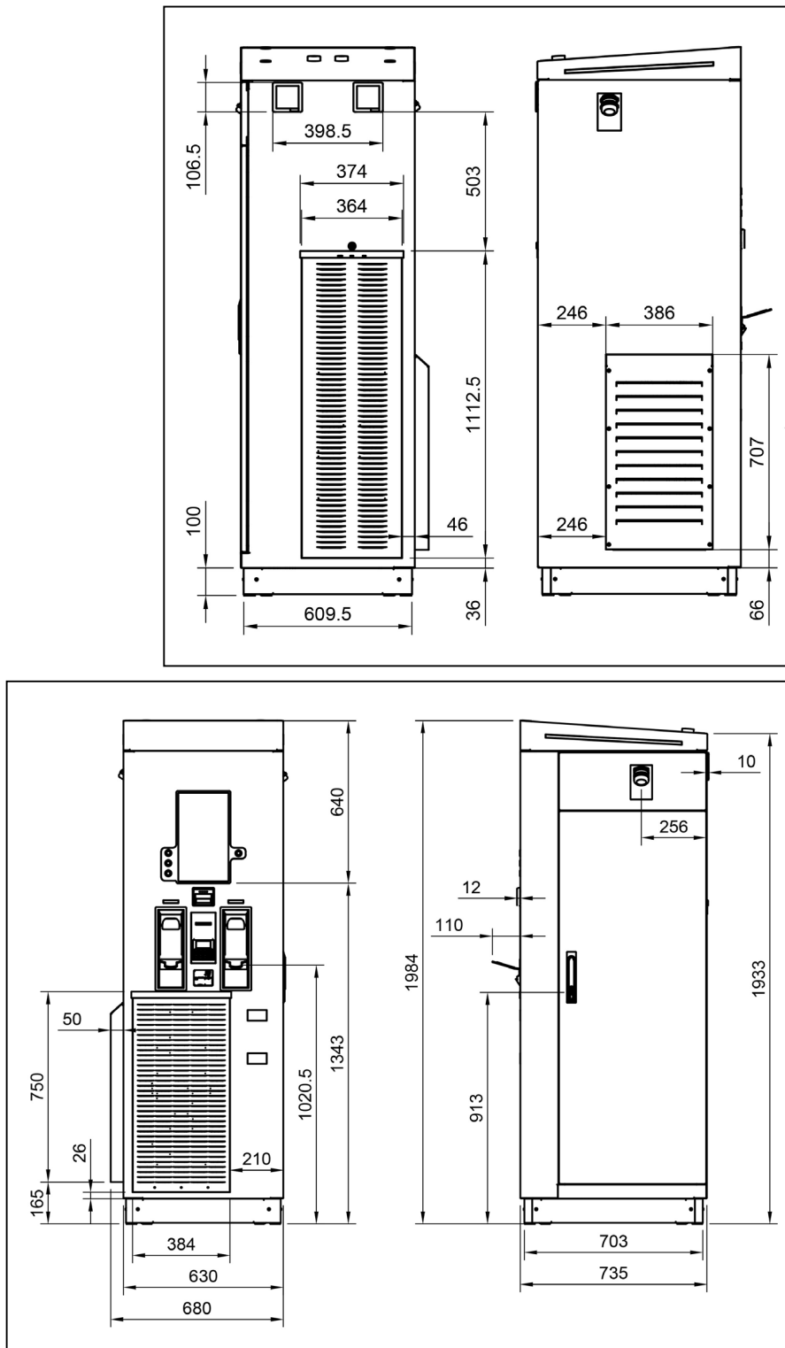
Abb. 52: Abmessungen
